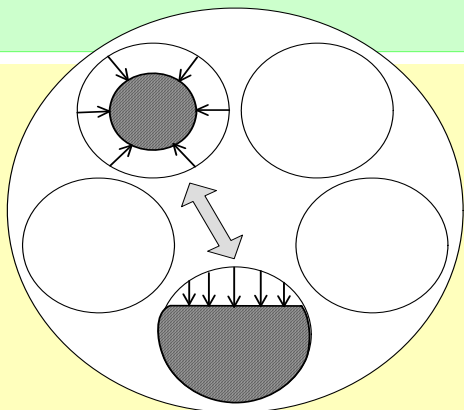
СВИТО равновесие
